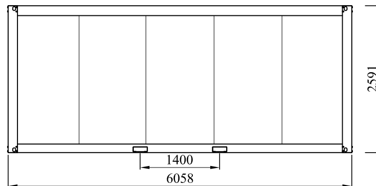
FASADA- D
