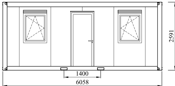
FASADA- A
